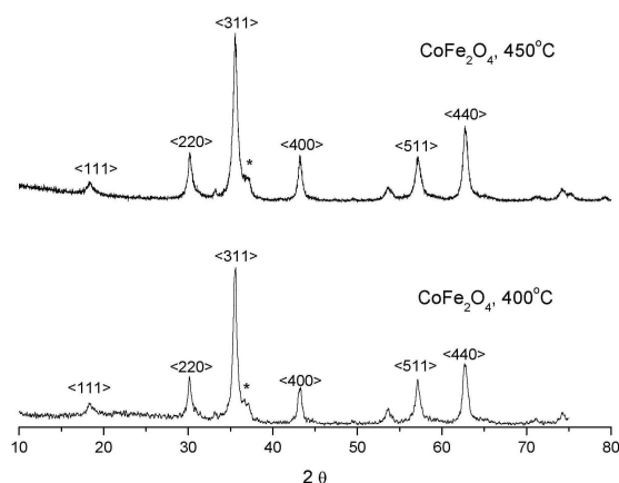
Fig. 3 - Padrões de difração de raios X das nanopartículas de CoFe 2 O 4 sintetizadas em 400 e 450°C em atmosfera de ar.
