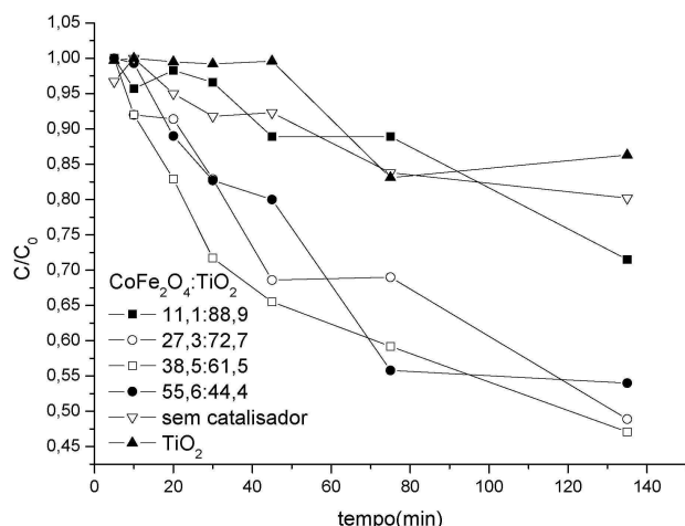
Fig. 5 - Perfil de degradação da atrazina em luz UV em função da adição de diferentes catalisadores.
