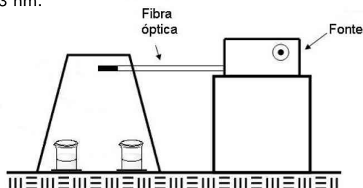
Fig. 1 - Esquema do aparato utilizado para fotodegradação do herbida atrazina com diferentes catalisadores
