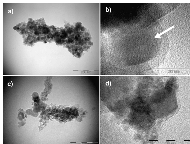
Fig. 4 - Imagens de microscopia eletrônica de transmissão de nanopartículas \text{CoFe}_2\text{O}_4@\text{TiO}_2 : a) aglomerado de nanopartículas de composição 11 \text{CoFe}_2\text{O}_4 :89 \text{TiO}_2 ; b) detalhe de nanopartícula de composição 11 \text{CoFe}_2\text{O}_4 :89 \text{TiO}_2 , mostrando uma partícula de \text{CoFe}_2\text{O}_4 ao centro de um encapsulamento; c) aglomerado de nanopartículas 55,5 \text{CoFe}_2\text{O}_4 :44,5 \text{TiO}_2 ; d) detalhe de nanopartícula 55,5 \text{CoFe}_2\text{O}_4 :44,5 \text{TiO}_2 mostrando encapsulamento.
