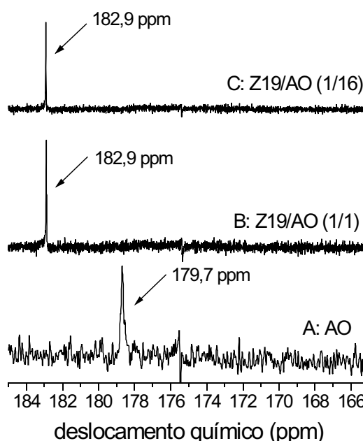
Figura 2: Espectros de RMN de ^{13}\text{C} de misturas de Z19 e ácido oléico marcado na carboxila com 99% de ^{13}\text{C} , em uma mistura etanol e água deuterada na razão 7/3. Espectro A: ácido oléico puro, espectro B: Z19/AO 1/1 e espectro C: razão Z19/AO 1/16. Os espectros foram adquiridos a 30°C.
