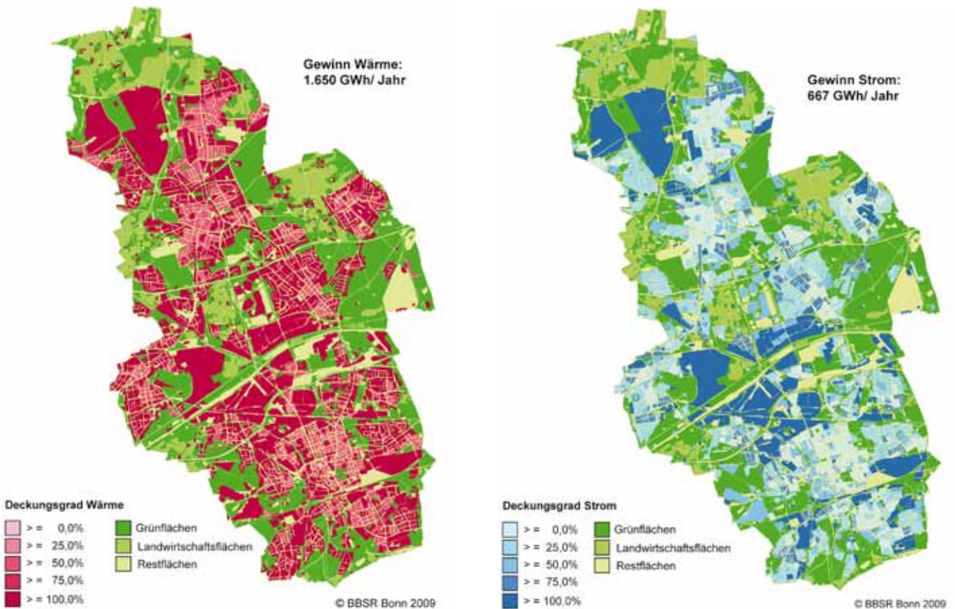
Karte 6 Wärmebereitstellung und Stromerzeugung nach Szenario VI in Gelsenkirchen
