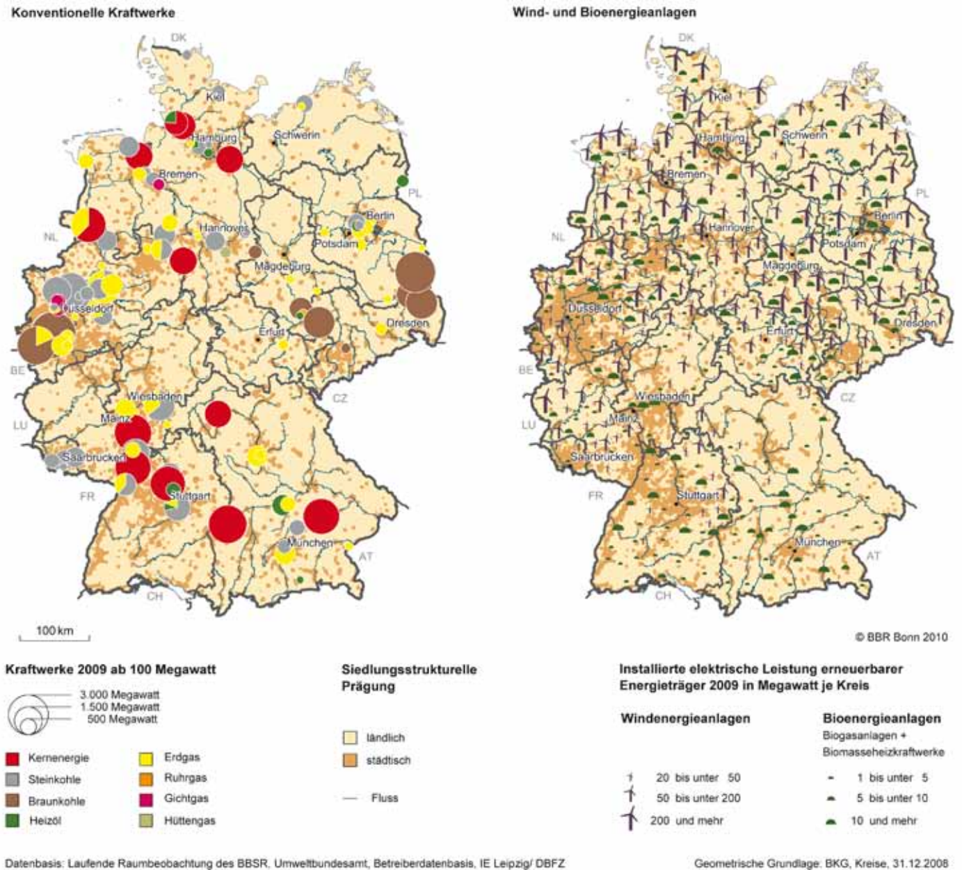
Karte 2 Konventionelle und erneuerbare Stromerzeugung im Raum
