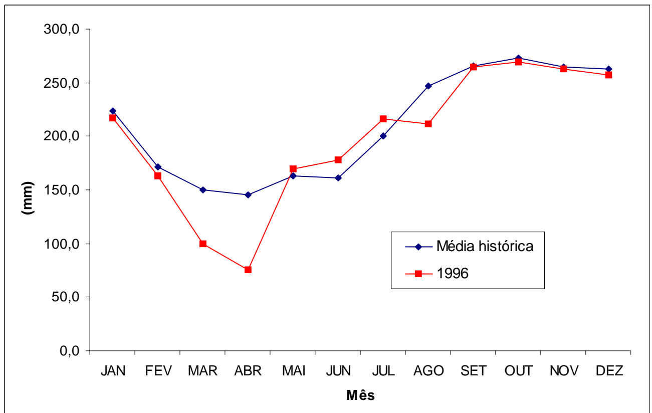
FIG. 4. Evaporação do tanque “Classe A”, totais mensais e anual em Fortaleza, 1996, comparada com a média histórica (1966-1996).
