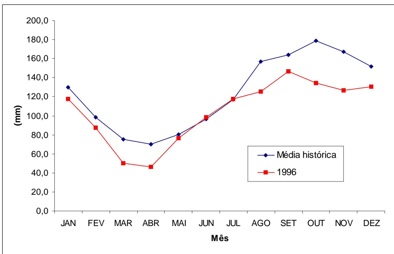
FIG. 5. Evaporação de Piche, totais mensais e anual em Fortaleza, 1996, comparada com a média histórica (1966-1996).
