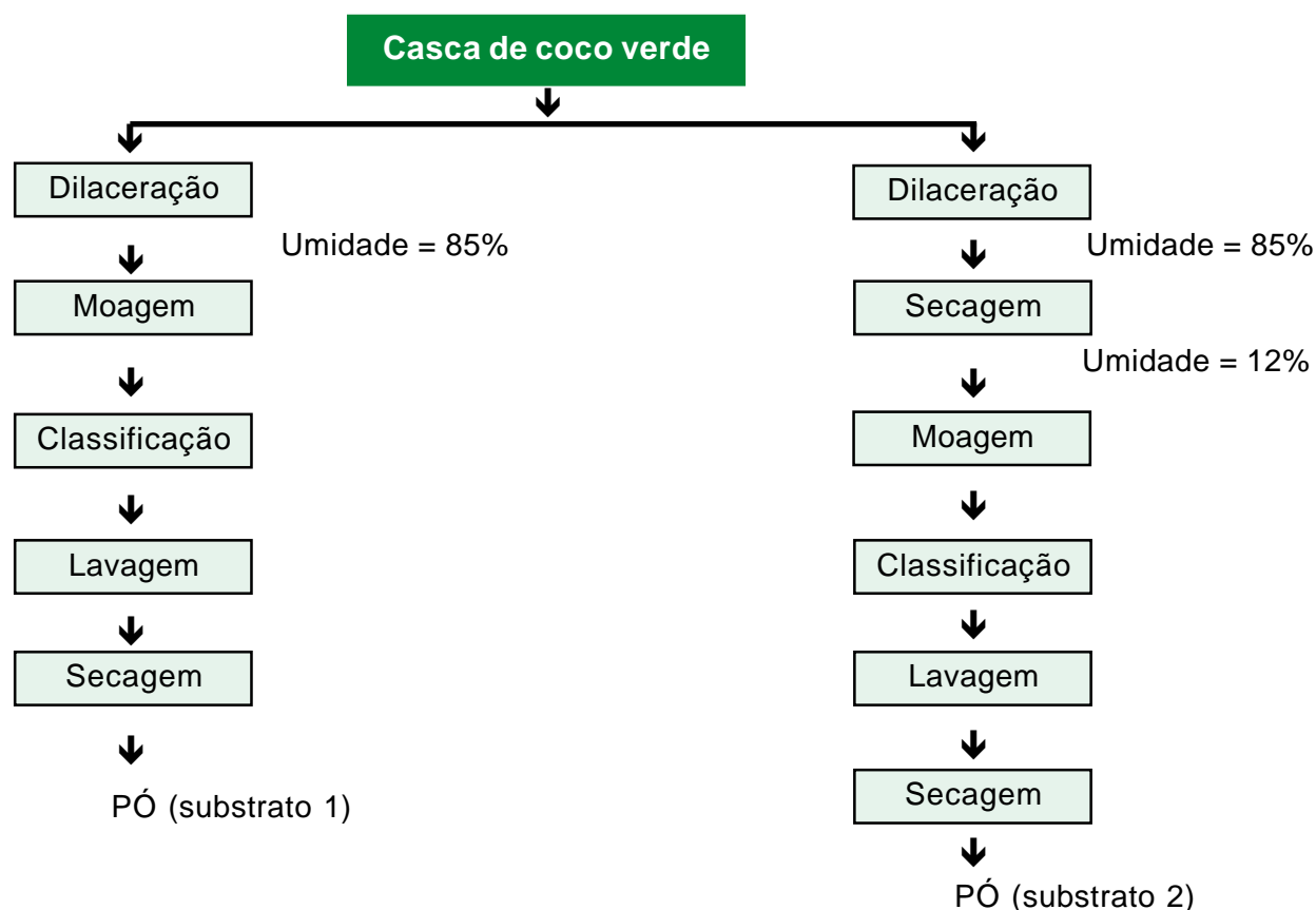
FIG. 1. Fluxograma das etapas de obtenção de pó de casca de coco verde.
