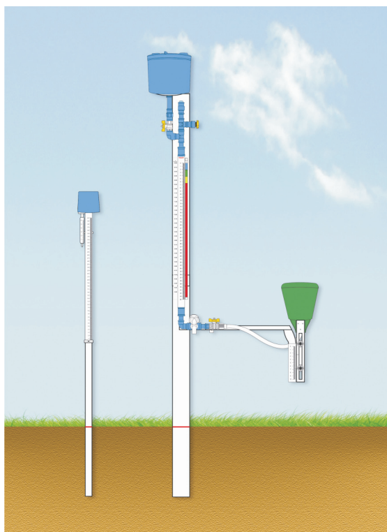
Fig. 1. Evaporímetro (direita) e Pluviômetro (esquerda) que compõem o Irrigâmetro.
