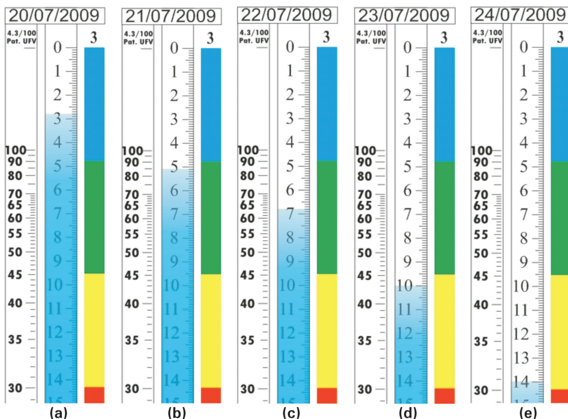
Fig. 3. Visualização das leituras diárias, no período de 20/07 a 24/07/2009, do Irrigâmetro instalado no Pivô Central.
