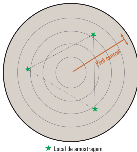
Fig. 2. Esquema de amostragem do solo em área a ser irrigada por pivô central.
