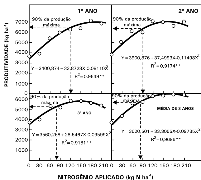
Fig. 1. Resposta do arroz irrigado à aplicação de nitrogênio em solo de várzea.
