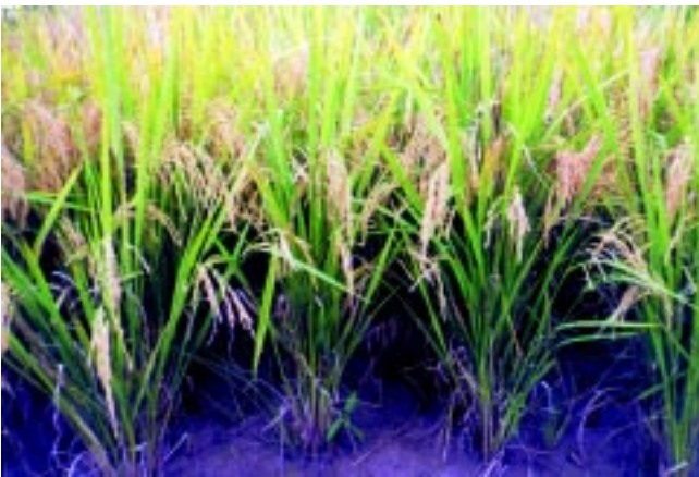
Fig. 3c. Aplicação 1/3 de N no plantio + 1/3 no perfilhamento ativo e 1/3 no inicial.
