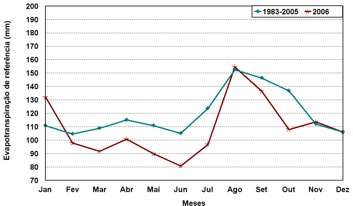
FIG. 3 Evapotranspiração de referência (1983-2005 e dados de 2006), estimada pelo método de Penman-Monteith, médias mensais, do município de Santo Antônio de Goiás-GO.
