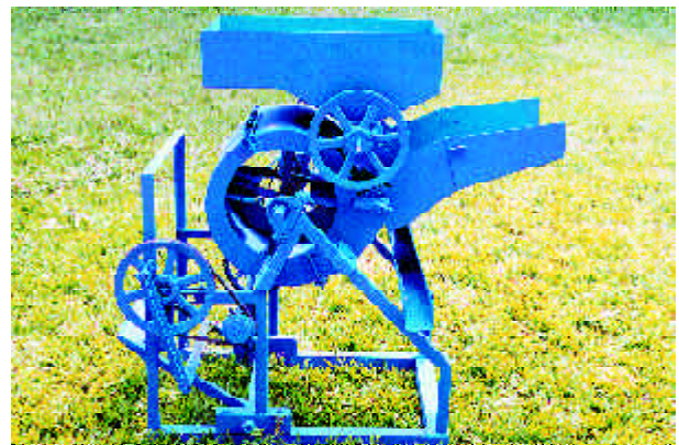
Fig. 1 Abanadora de sementes com ventilador acionado a pedal.
