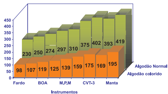
Fig. 1. Comportamento do algodão de coloração normal e colorido nos instrumentos de abertura e de limpeza, do fardo à manta.
