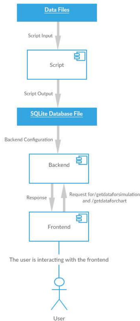
Figure 13 - A komponensek áttekintése
