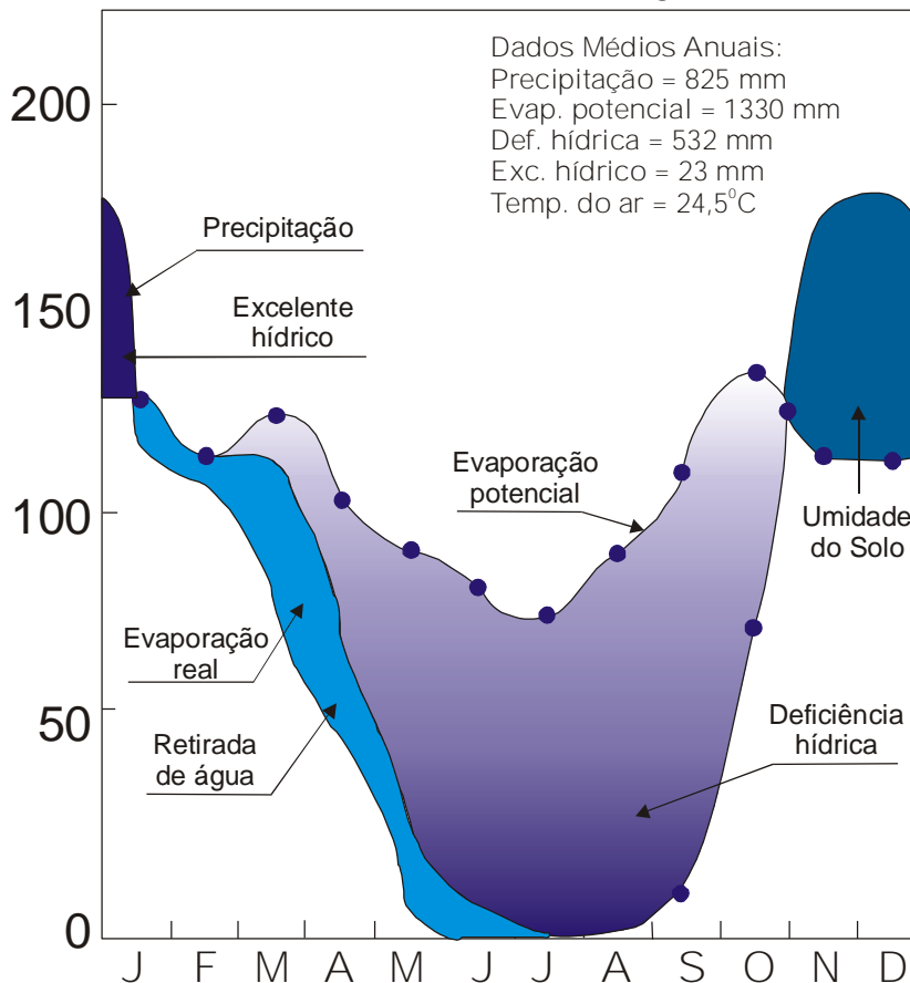
Fig. 1. Balanço hídrico pelo método de Thornthwaite & Mather, 1955. Fonte: Antunes (1978).
