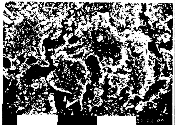
Fotos 3 y 4: Imágenes MEB, mostrando el daño causado por el líquen Staurothele frustulenta .
