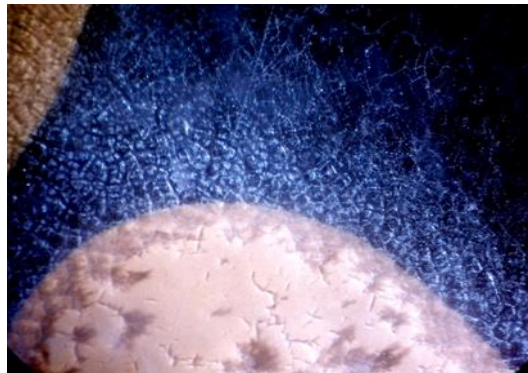
FIGURA 10 - Macrofotografia de obra em acrílico que apresenta Crazing tipo H –Aleatória Ramificada com sinais de despolimerização. Fonte: FRANÇA, 2008
