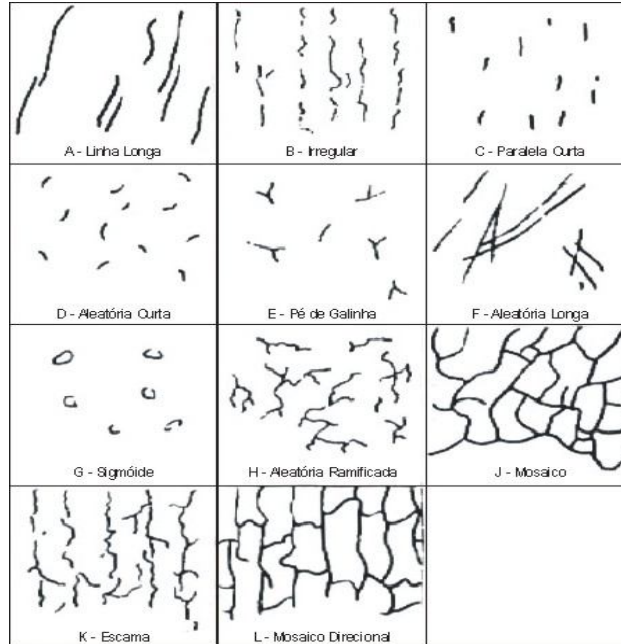
FIGURA 4 – Padrões de referência para a identificação e comparação de cracking . Fonte: FAZANO, 1995
