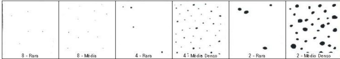
FIGURA 7 – Padrões de tamanho e freqüência de empolamento ( blister ). Fonte: FAZANO, 1995
