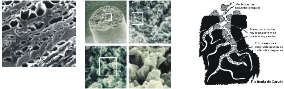
FIGURA 8 – Fotografias ampliadas da superfície de uma partícula de carvão ativado e esquema de adsorção das partículas pelos poros. Fonte: FRANÇA, 2008.
