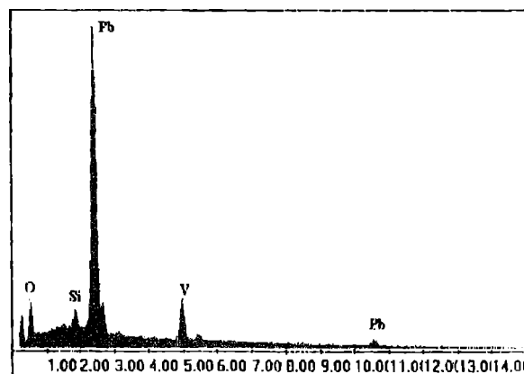
Figura 5b. EDAX correspondiente al cristal prismático piramidal de la figura 5a.
