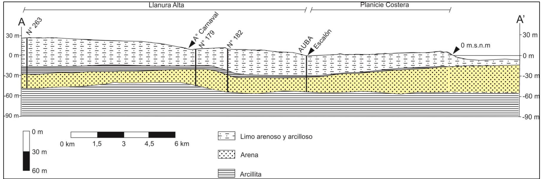
Figura 3. Sección geológica AA' en sentido NE-SO.
