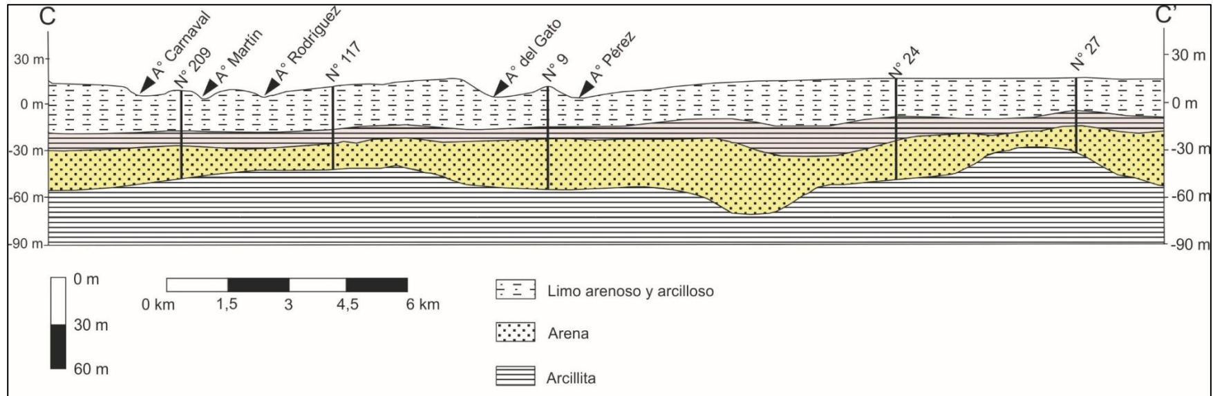
Figura 5. Sección geológica CC' en sentido NO-SE.
