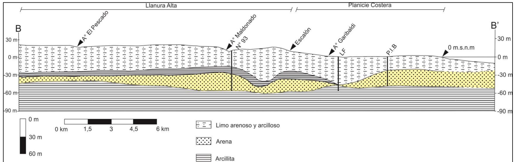
Figura 4. Sección geológica BB' en sentido NE-SO.
