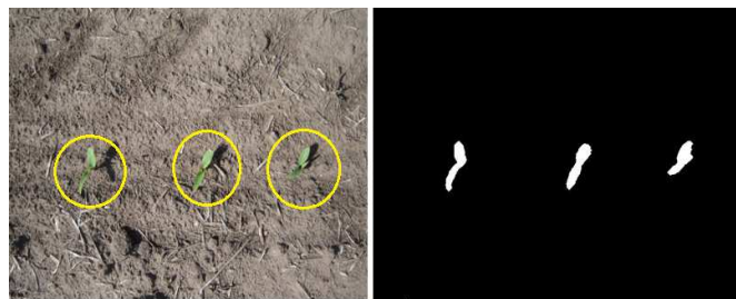
Fig. 9. Corrida algoritmo de conteo (altura: 1 m).
