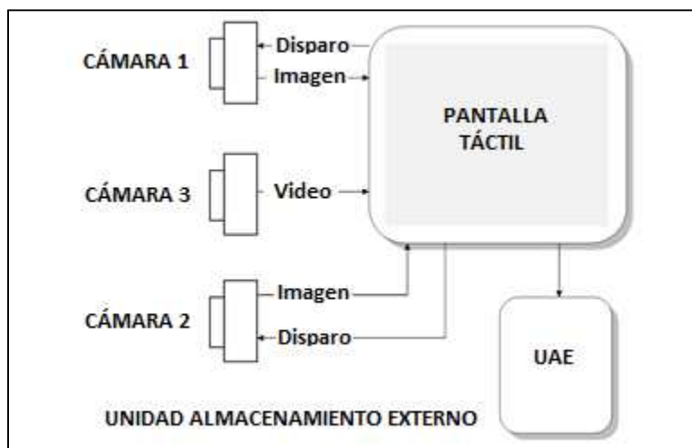
Fig. 5. Interconexión de dispositivos, circuito de disparo.
