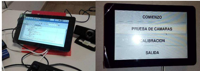
Fig. 8. Raspberry utilizada como UC en pruebas en nuestro laboratorio, e interfaz de usuario.
