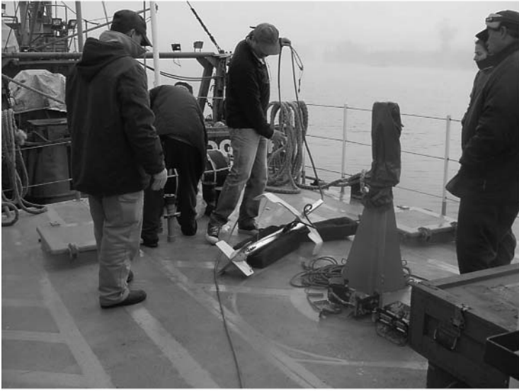
Figura 3: Equipo de sonar lateral y muestreador Snapper sobre la borda de la lancha.
