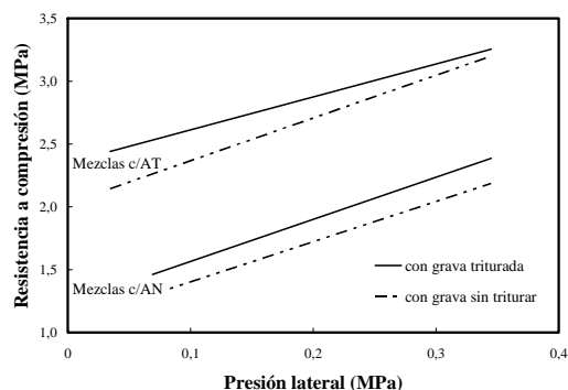
Figura 2.3: Ensayo triaxial de mezclas asfálticas con arena natural (AN) y arena triturada (AT). (adaptado de Gray, 1964).
