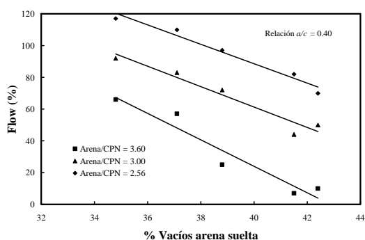
Figura 3.12: Relación entre la fluidez de morteros, con diferentes proporciones agregado/cemento, y el contenido de vacíos de la mezcla de arena suelta. (experiencias del autor, R^2=0.93-0.97 )
