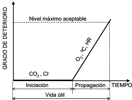
Figura 4.33: Modelo simplificado de deterioro del acero en el hormigón.
