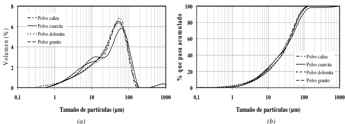
Figura 5.4: Granulometría del polvo de roca: en % que pasa parcial (a) y acumulado (b)
