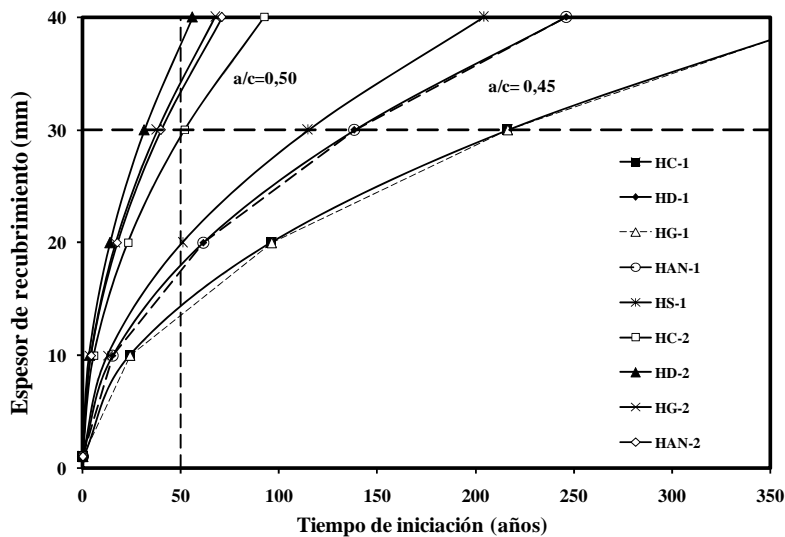
Figura 8.7: Tiempo de iniciación para diferentes hormigones empleando el modelo de la Instrucción EHE-2008.
