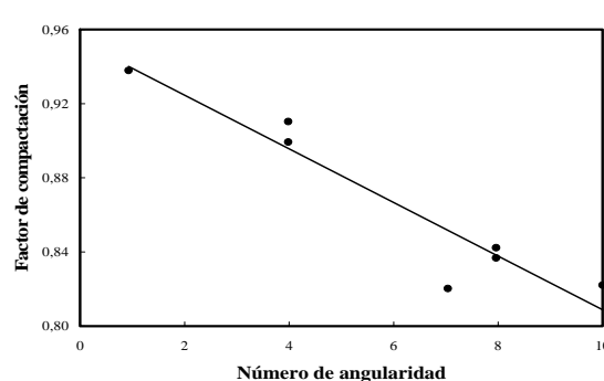
Figura 3.13: Relación entre el número de angularidad del agregado grueso y el factor de compactación del hormigón (adaptado de Shergold, 1953).
