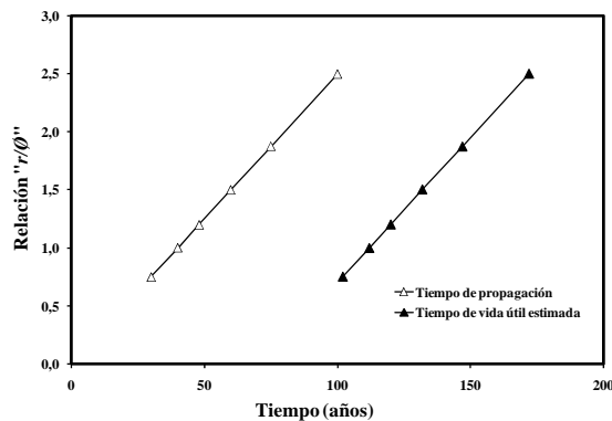
Figura 8.5: Influencia de la relación “ C/\varnothing ” sobre los tiempos de propagación y de vida útil estimada (EHE, 2008).
