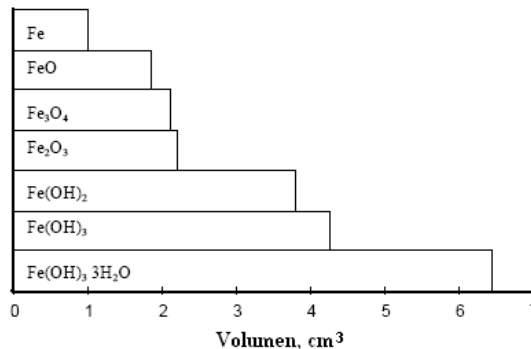
Figura 4.36: Volumen de óxido e hidróxidos de hierro, respecto al volumen de hierro corroído.
