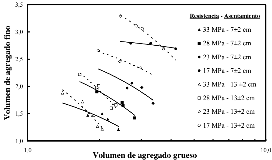
Figura VII.5: Nomograma para la dosificación por volumen, en base a un volumen de cemento, para dos rangos de consistencias ( R^2=0.71-0.99 ).
