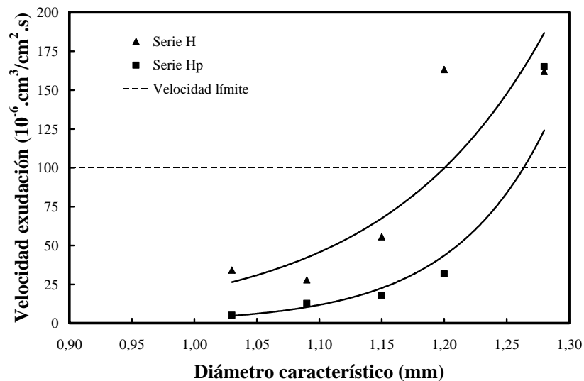
Figura 6.13: Relación entre el diámetro característico de la arena y la velocidad exudación de las Series H y Hp ( R^2=0.81-0.96 ).
