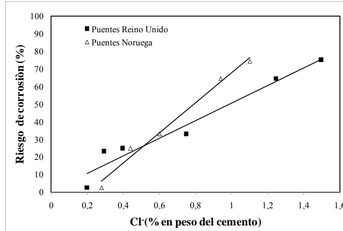
Figura 4.40: Relación entre el riesgo de corrosión y el contenido de cloruros (Villagrán, 2012).
