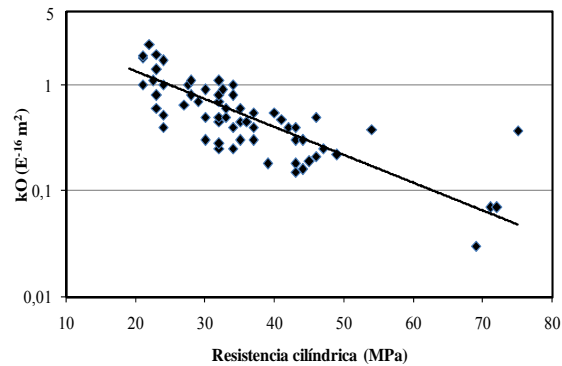
Figura 4.30: Permeabilidad al oxígeno ( kO ) vs resistencia a la compresión.
