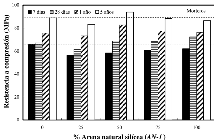
Figura 7.10: Resistencia a compresión del mortero en función del contenido de arena natural sílicea.
