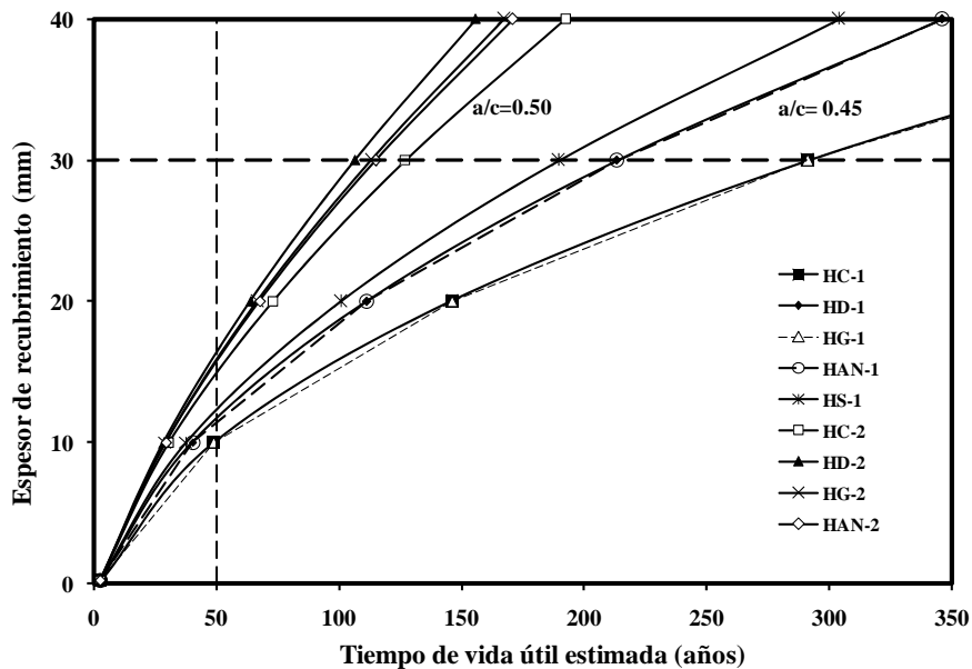
Figura 8.8: Tiempo de vida útil estimada para diferentes hormigones según el modelo de la Instrucción EHE-2008.
