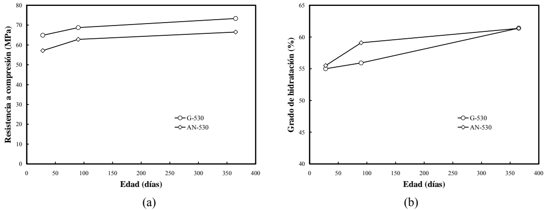
Figura 7.11: Desarrollo de la resistencia (a) y del grado de hidratación (b) de las mezclas AN-530 y G-530.
