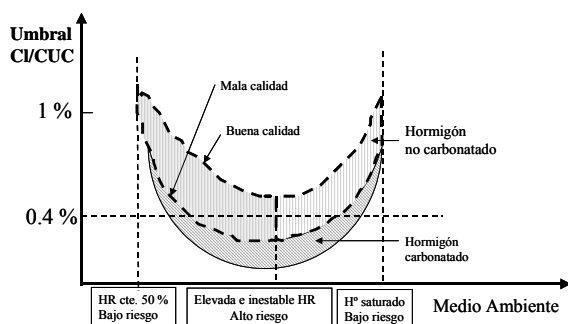
Figura 4.38: Umbral de cloruros en función de la calidad del hormigón y la HR (Feliú, 1988).
