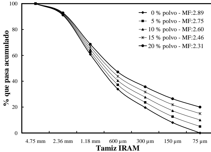
Figura 5.7: Modificación de la granulometría del agregado fino por la incorporación de polvo.
