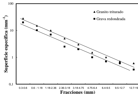
Figura 3.21: Relación entre la superficie específica y el tamaño de la partícula. (adaptado de Neville, 1988).
