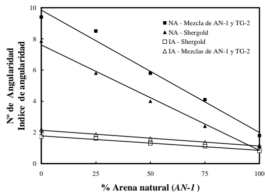
Figura 3.14: Número e índice de angularidad para mezclas de arenas triturada y natural (experiencias del autor; R^2=0.98-0.99 ).
