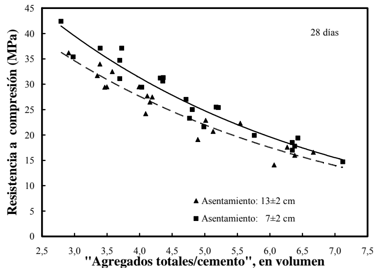
Figura VII.4: Resistencia a compresión de hormigones con arenas trituradas graníticas vs. la relación agregado/cemento ( R^2=0.90-0.94 ).
