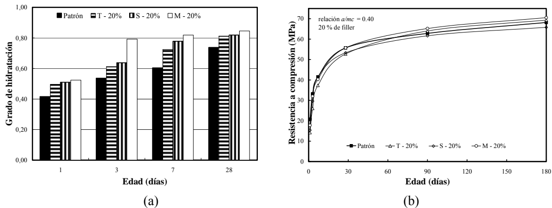
Figura 4.11: Grado de hidratación (a) y resistencia a compresión de pastas con 20 % de filler calizo (b). (adaptado de Bonavetti, 1998) (T: 360 m 2 /kg – S: 710 m 2 /kg – M: 1020 m 2 /kg)
