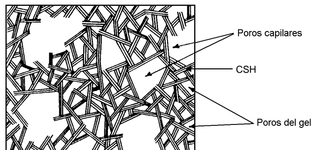
Figura 4.7: Esquema de la pasta de cemento hidratada según el modelo de Powers (Soroka, 1979).
