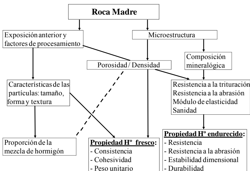
Figura 4.16: Esquema de la influencia de la microestructura, exposición anterior y factores de procesamiento de los agregados sobre las propiedades del hormigón (adaptado de Mehta, 1993).
