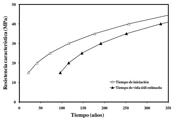
Figura 8.4: Influencia de la resistencia del hormigón sobre los tiempos de iniciación y de vida útil estimada, para \varnothing = 16 mm y 30 mm de recubrimiento (EHE, 2008).
