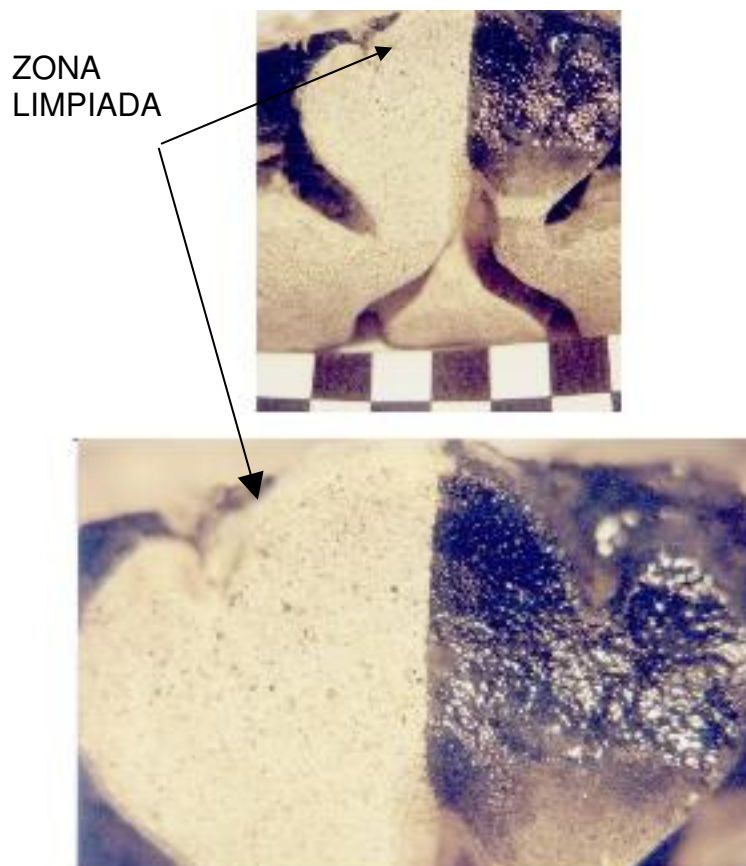
Figura 1: Limpieza con láser de una moldura de concreto
