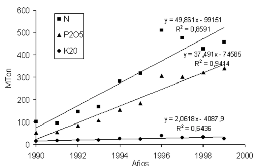
Figura 1. Tendencias en el consumo de nitrógeno (N), pentóxido de fósforo ( \text{P}_2\text{O}_5 ) y dióxido de potasio ( \text{K}_2\text{O} ) (millones de toneladas) para el total del país en el período 1990-1999. Elaboración propia sobre la base de datos de FAO (2002).
