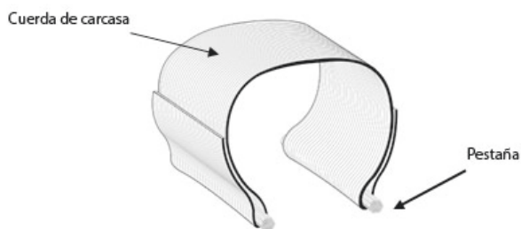
Detalle de la muestra de alambre tomada de zona pestaña
