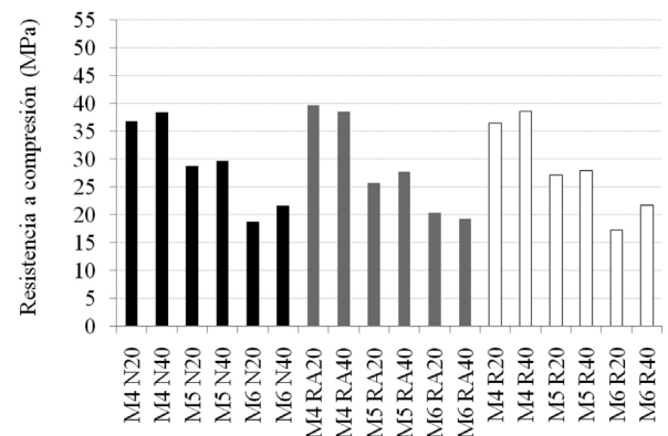
Figura 8. Resistencia a compresión a 7 días.
