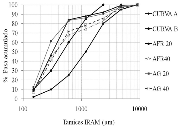
Figura 2. Granulometrías de los agregados.
