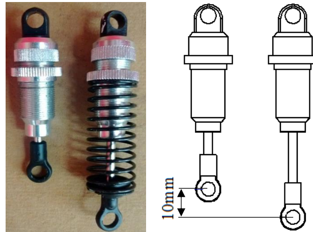
Figura 2. Amortiguador-espiral HG.
