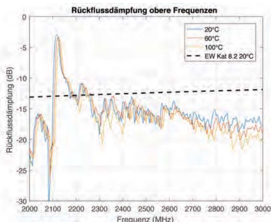
Abb. 5: Messung Rückflussdämpfung höherer Frequenzen in Abhängigkeit von der Umgebungstemperatur (farbige Kurven) und Extrapolation (EW) oberhalb 2 GHz
