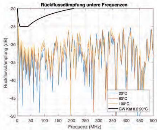
Abb. 4: Messung Rückflussdämpfung unterer Frequenzen in Abhängigkeit von der Umgebungstemperatur (farbige Kurven) und Grenzwertkurve (GW) für 20 °C
