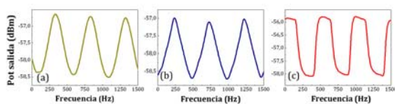
Fig. 3. Modulaciones medidas en \lambda_{NOMOD} .
