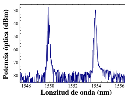
Fig. 2. Espectro óptico del EDFRL con una modulación de 2KHz aplicada a \lambda=1554 nm.
