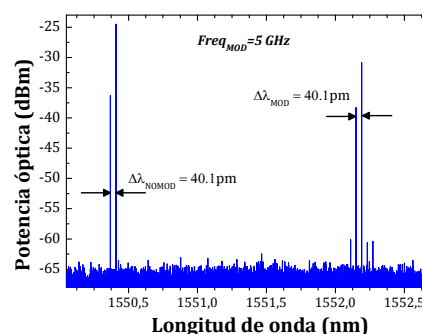
Fig. 4. Espectro óptico al aplicar una modulación de 5GHz en \lambda=1552.2 nm.
