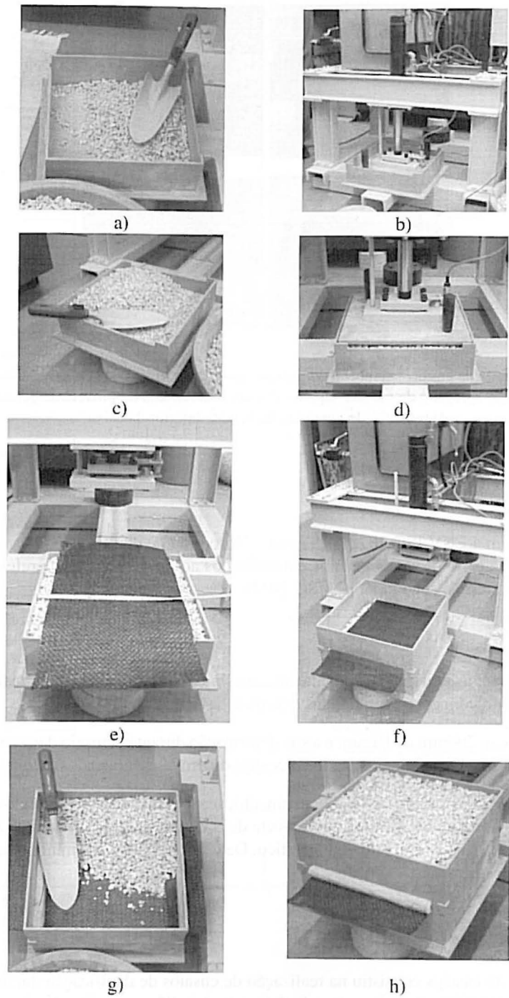
Fig. 12 – Método de ensaio: a) colocação da 1ª camada de agregado na metade inferior da caixa; b) compactação da 1ª camada de agregado; c) colocação da 2ª camada de agregado na metade inferior da caixa; d) compactação da 2ª camada de agregado; e) colocação do provete de geossintético; f) colocação da metade superior da caixa; g) enchimento da metade superior da caixa com agregado solto; h) vista da caixa antes do início do ensaio.
