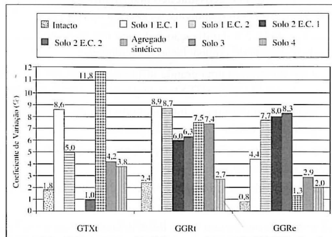
Fig. 19 – Ensaio in situ e de laboratório – coeficiente de variação da resistência à tracção.
