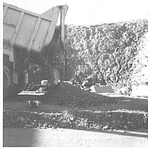
d) deposição da 2ª camada de solo
