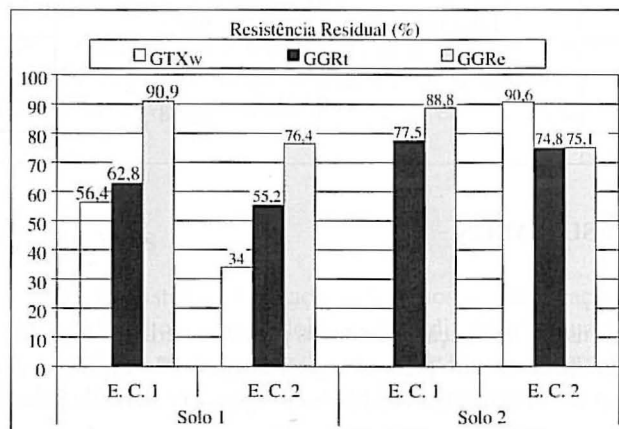
Fig. 14 – Ensaios in situ – resistência residual.
