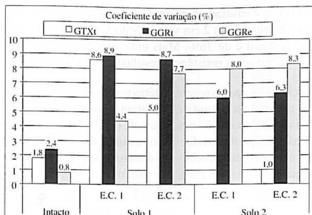
Fig. 15 – Ensaio in situ – coeficiente de variação da resistência à tracção.
