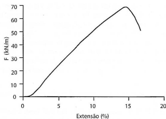
Fig. 1 – Comportamento à tracção do geotêxtil GTXt.
