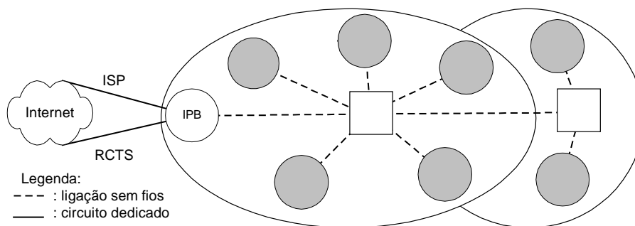
Fig. 2 – Topologia simplificada da solução baseada em ligações sem fios.
