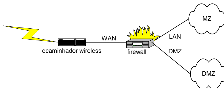
Fig. 4 – Topologia local típica.
