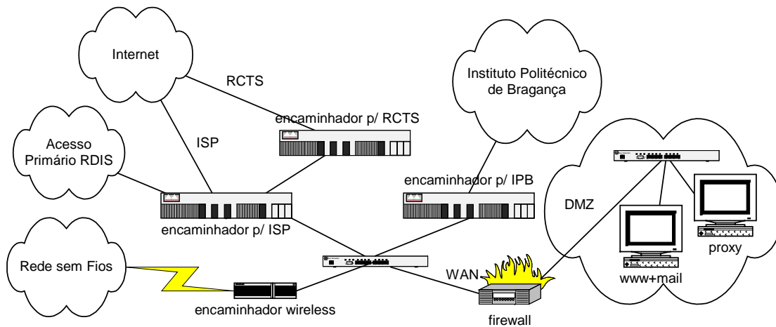
Fig. 5 – Topologia no ponto de acesso à Internet (IPB).
