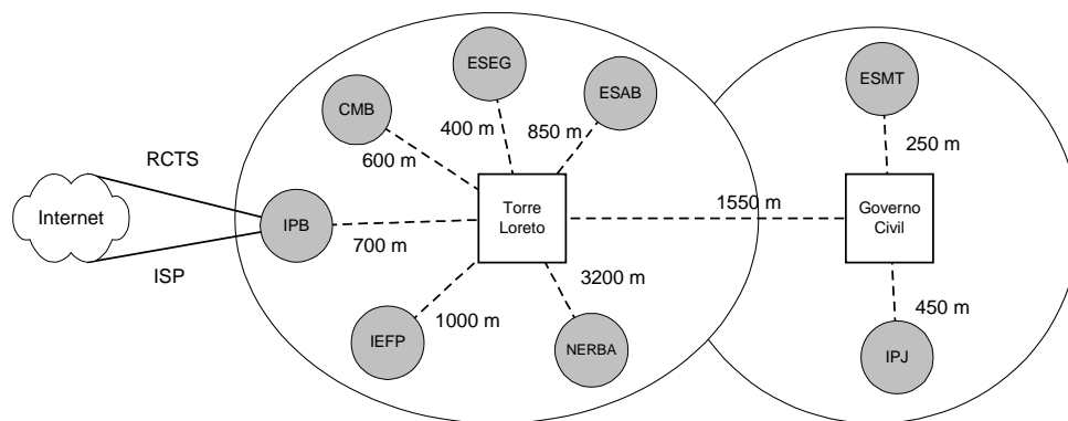
Fig. 3 – Topologia à escala metropolitana.
