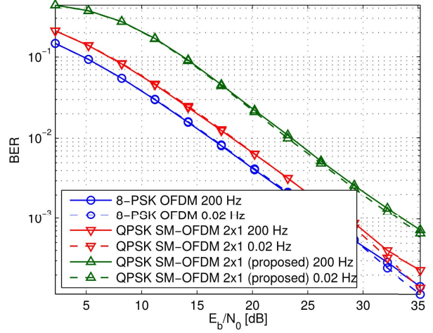
Fig. 4. BER
