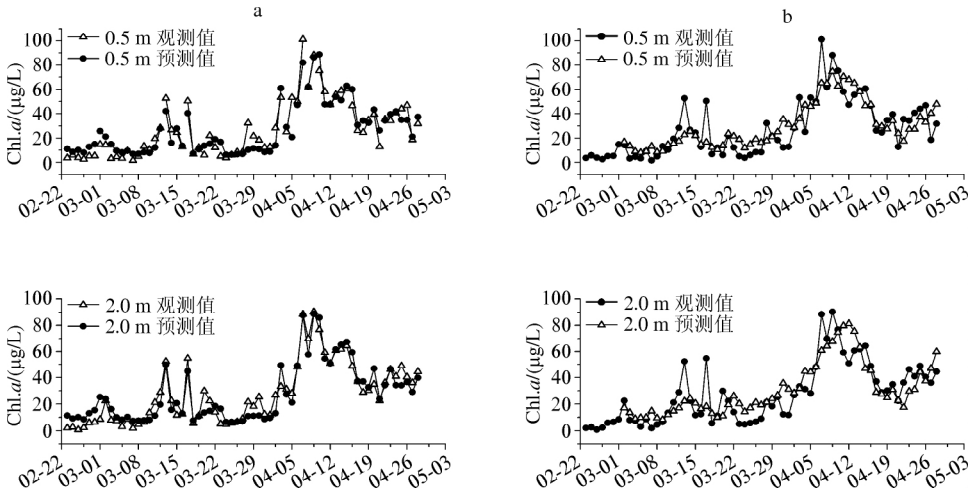
图 3 香溪河库湾藻类水华期间叶绿素 a 浓度预测结果( a: 实时 b: 提前 7 d)
