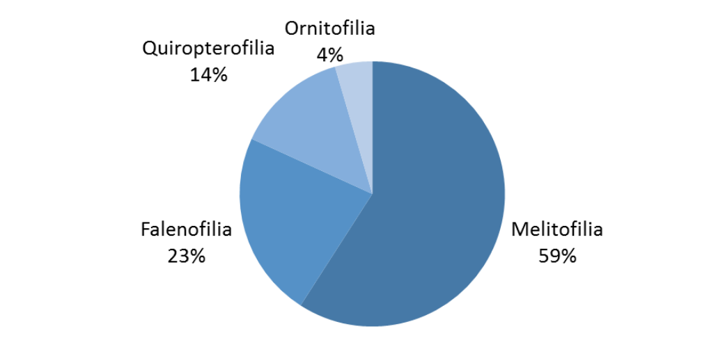
Grafico 1: Síndromes de polinização
