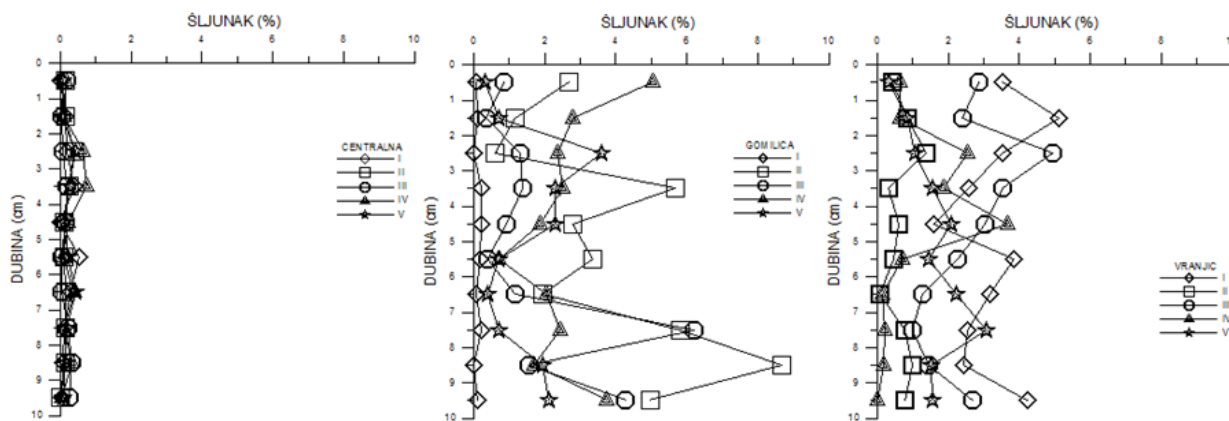
Slika 45. Udio čestica veličina šljunka (%) u pet uzorkovanja u jezgrama istraživanih postaja
