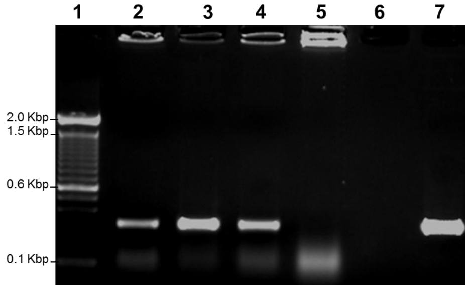
Figure 20. Detection of the melittin gene in B subtilis transformed with pHT01-Mel by PCR. 100bp DNA marker (lane 1); B.subtilis 1012 pHT01-Mel (lane 2); B.subtilis 168 pHT01-Mel (lane 3); pHT01-Mel DNA (lane 4, + control); B.subtilis -pHT01- (lane 5,- control); PCR-Blank (lane 6, no DNA); pHT01-Mel DNA, colony (lane 7, + control).
