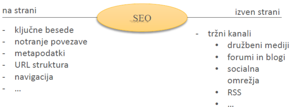
Slika 2.1: SEO-razdelitev zahtev
