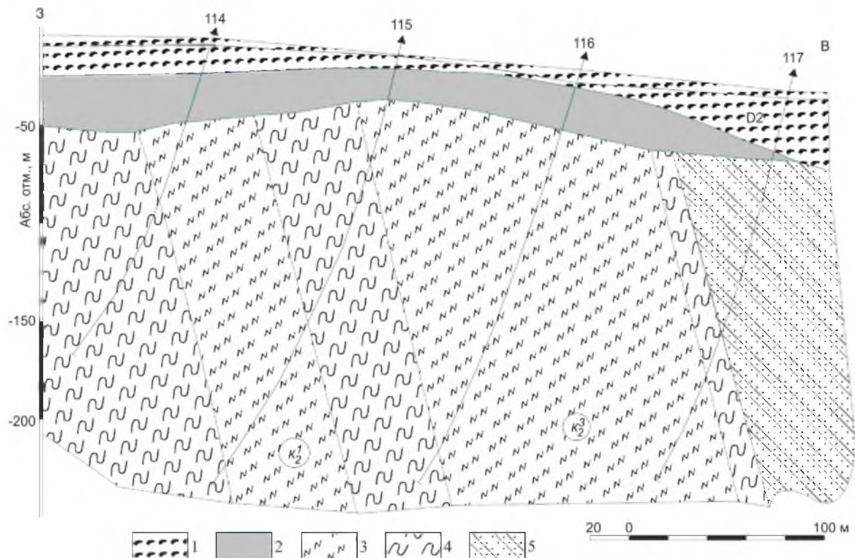
Рис. 2. Геологический разрез коры выветривания по профилю X Осколецкого месторождения (по И.И. Никулину и А.Д. Савко [2015]): 1 – девонские глины и аргиллиты; 2 – остаточная кора выветривания; 3 – железистые кварциты; 4 – сланцы; 5 – карбонатные метаморфические породы
