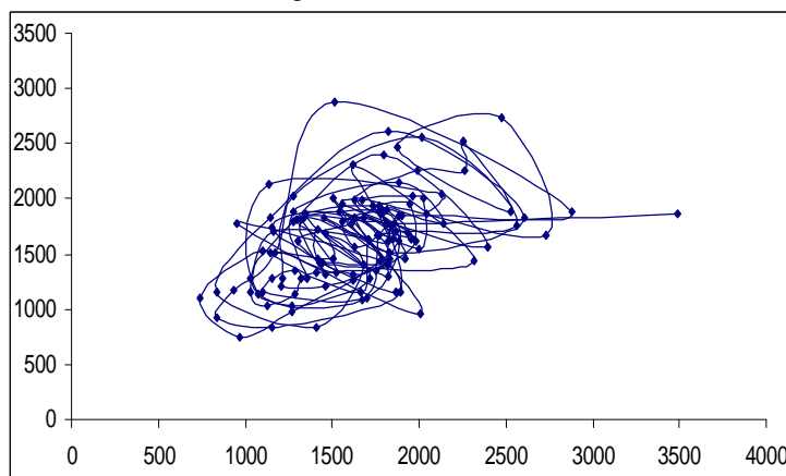
Рисунок 1. Фазовый портрет временного ряда помесечного количества заболевших ОРЗ детей
