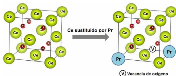
Figura 3. Celda unitaria de \text{CeO}_2 y la variación de la celda unitaria durante el proceso de dopaje (Elaboración propia utilizando el software VESTA).
