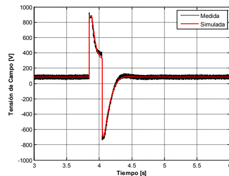
Fig. 4. Pulso +15\% , 0,2\text{ s} . Tensión de Campo.
