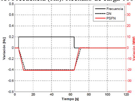
Fig. 17. Escalón 0,2 Hz. Var. de Frecuencia con RPF. Fig. 18. Escalón 0,2 Hz. Potencia Activa con RPF.
