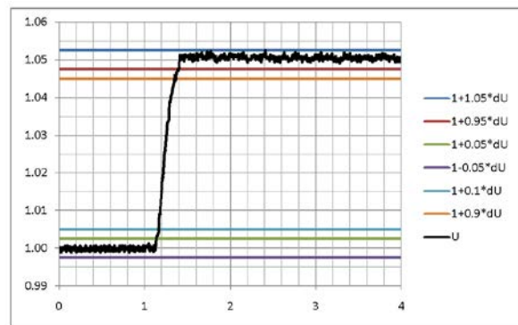
Fig. 2. Tensión Terminal. Respuesta a Escalón +5\% en Referencia Tensión.
