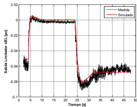
Fig. 8. UEL. Pulso -3 %, 20 s. Salida del Limitador.
