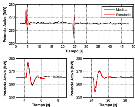
Fig. 11. Pulso +3 %, 20 s. Potencia Activa. Con PSS
