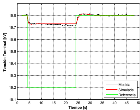
Fig. 7. UEL. Pulso -3 %, 20 s. Tensión Terminal.
