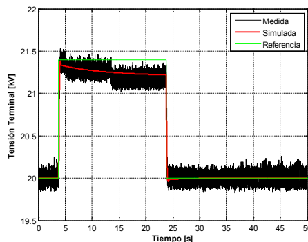
Fig. 5. V/Hz. Pulso +7\% , 20\text{ s} . Tensión Terminal.
