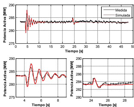
Fig. 9. UEL. Pulso -3 %, 20 s. Potencia Activa.
