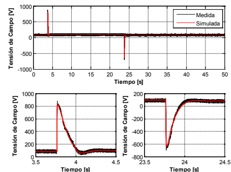
Fig. 6. V/Hz. Pulso +7\% , 20\text{ s} . Tensión de Campo.
