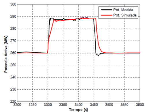
Fig. 20. Escalón 2 Hz. Potencia Activa con RPF.
