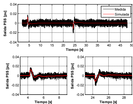
Fig. 12. Pulso +3 %, 20 s. Salida PSS. Con PSS.
