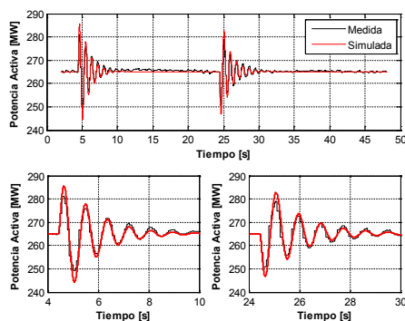
Fig. 13. Pulso +3 %, 20 s. Potencia Activa. Sin PSS.
