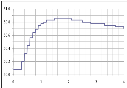
Fig. 15. Frecuencia (Hz). Rechazo de carga 100 MW.
