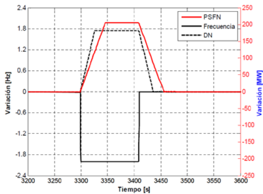
Fig. 19. Escalón 2 Hz. Var. de Frecuencia con RPF.
