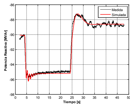
Fig. 10. UEL. Pulso -3 %, 20 s. Potencia Reactiva.
