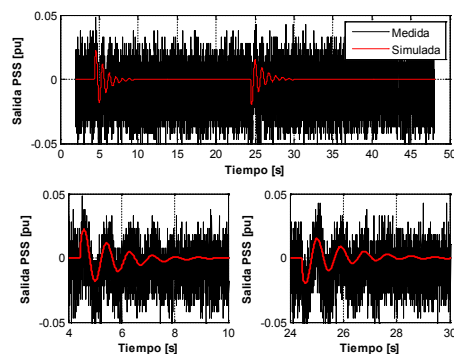
Fig. 14. Pulso +3 %, 20 s. Salida PSS. Sin PSS.
