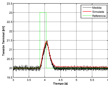
Fig. 3. Pulso +15\% , 0,2\text{ s} . Tensión Terminal.
