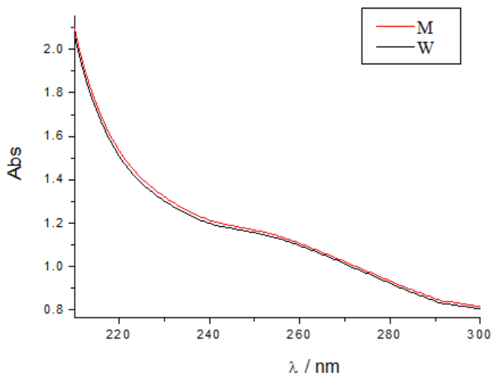
Slika 38. Usporedba apsorpcijskih spektara otopina RNA divljeg tipa (crno) i RNA sa mutacijom (crveno).
