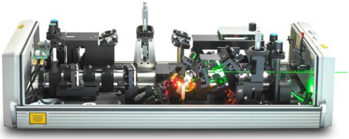
Slika 21: Unutrašnjost Tsunami lasera i preuzeta je iz [36]. Vidi se ulazni zeleni snop s desne strane (tipično 532 nm).
