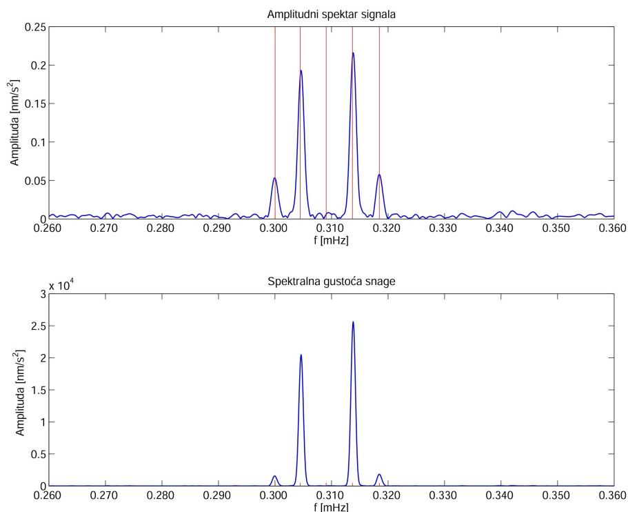
Slika 3.7 Amplitudni spektar i spektralna gustoća snage za signal nakon potresa u području Tohoku iz 2011. godine za postaju BFO (Njemačka). Prikazan je 0S_2 mod i razdvajanje moda na njegove singlete. Na spektru nije pobuđen m = 0 singlet.
