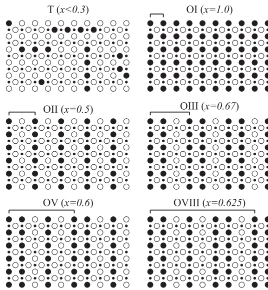
Slika 5.3: Periodični uzorci i imena pripadnih faza Cu–O lanaca u YBCO kristalu. T označava nasumičan razmještaj kisika (tetragonalna simetrija), a O različite ortoromske faze Cu–O lanaca s tipičnim dopiranjem za pojedinu fazu. o su prazne, a • popunjene pozicije kisika.
