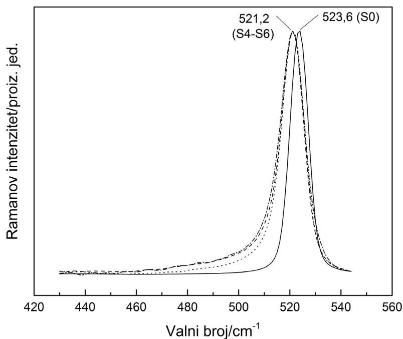
Slika 60. Normirani Ramanovi spektri uzoraka poroznog silicija S_4 (crtice), S_5 (točkice), S_6 (crtica – točkica) i kristalnog silicija S_0 (puna linija).
