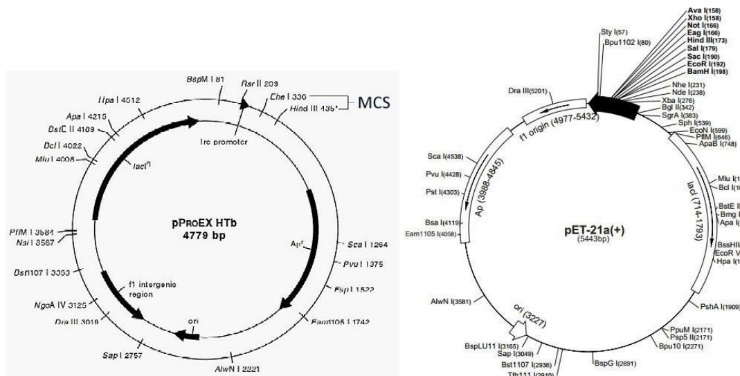
Slika 3-1. Mape vektora pProEx-HTb (lijevo) i pET-21a (desno). Skraćenica MCS stoji za eng. multi-cloning site (višestruko mjesto za kloniranje), Ap r je gen bla s kojeg se sintetizira enzim odgovoran za rezistenciju na ampicilin, ori mjesto ishodišta replikacije. Duljina (u parovima baza) dana je ispod imena plazmida.
