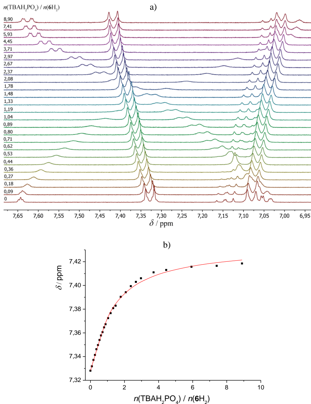
Slika 70. a) ^1\text{H} NMR titracija 6\text{H}_2 ( c = 6,10 \times 10^{-4} \text{ mol dm}^{-3} ) s \text{TBAH}_2\text{PO}_4 ( c = 9,49 \times 10^{-3} \text{ mol dm}^{-3} ) u \text{DMSO-}d_6 pri (25,0 \pm 0,1) \text{ }^\circ\text{C} . b) Ovisnost kemijskog pomaka \text{H}_a protona tijekom ^1\text{H} NMR titracije s \text{TBAH}_2\text{PO}_4 o množinskom omjeru n(\text{TBAH}_2\text{PO}_4) / n(6\text{H}_2) . ■ izmjerene vrijednosti, — izračunane vrijednosti.
