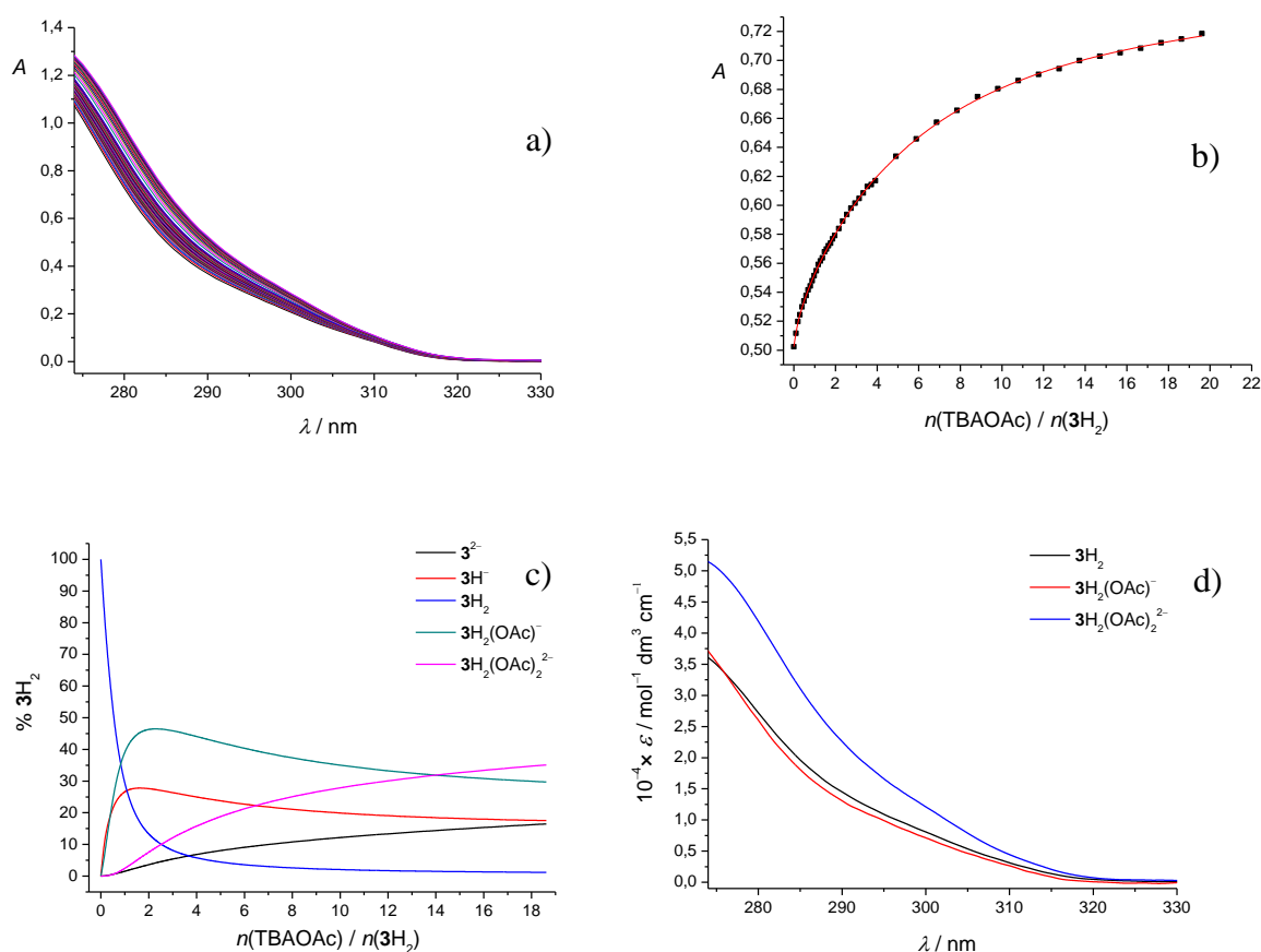
Slika 39. a) Spektrofotometrijska titracija 3H_2 ( c = 2,90 \times 10^{-5} mol dm -3 ) s TBAOAc ( c = 1,32 \times 10^{-3} mol dm -3 ) u DMSO. Spektri su korigirani za razrjeđenje. l = 1 cm, (25,0 \pm 0,1) °C. b) Ovisnost apsorbancije otopine 3H_2 pri 285 nm o množinskom omjeru n(\text{TBAOAc}) / n(3H_2) . ■ izmjerene vrijednosti, — izračunane vrijednosti. c) Distribucija pojedinih vrsta tijekom titracije otopine 3H_2 s TBAOAc. d) Karakteristični UV spektri spoja 3H_2 i njegovih kompleksa s acetatom.
