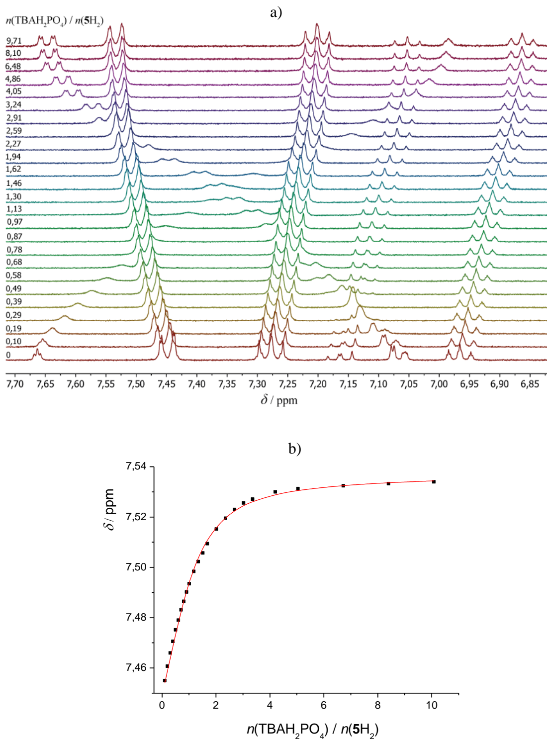
Slika 69. a) ^1\text{H} NMR titracija 5\text{H}_2 ( c = 6,00 \times 10^{-4} \text{ mol dm}^{-3} ) s \text{TBAH}_2\text{PO}_4 ( c = 1,02 \times 10^{-2} \text{ mol dm}^{-3} ) u \text{DMSO-}d_6 pri (25,0 \pm 0,1) ^\circ\text{C} . b) Ovisnost kemijskog pomaka \text{H}_d protona tijekom ^1\text{H} NMR titracije s \text{TBAH}_2\text{PO}_4 o množinskom omjeru n(\text{TBAH}_2\text{PO}_4) / n(5\text{H}_2) . ■ izmjerene vrijednosti, — izračunane vrijednosti.
