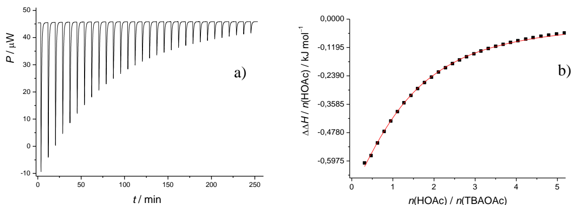
Slika 21. a) Mikrokalorimetrijska titracija otopine TBAOAc ( c = 5 \times 10^{-3} \text{ mol dm}^{-3} ) s HOAc ( c = 0,110 \text{ mol dm}^{-3} ) u DMSO pri 25 °C. b) Ovisnost sukcesivne promjene entalpije o množinskom omjeru n(\text{HOAc}) / n(\text{TBAOAc}) ; ■ izmjerene vrijednosti, — izračunane vrijednosti.
