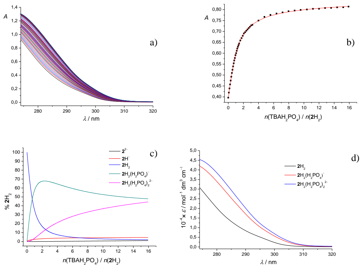
Slika 44. a) Spektrofotometrijska titracija 2\text{H}_2 ( c = 3,00 \times 10^{-5} \text{ mol dm}^{-3} ) s \text{TBAH}_2\text{PO}_4 ( c = 1,11 \times 10^{-3} \text{ mol dm}^{-3} ) u DMSO. Spektri su korigirani za razrjeđenje. l = 1 \text{ cm} , (25,0 \pm 0,1) \text{ }^\circ\text{C} . b) Ovisnost apsorbancije otopine 2\text{H}_2 pri 285 nm o množinskom omjeru n(\text{TBAH}_2\text{PO}_4) / n(2\text{H}_2) . ■ izmjerene vrijednosti, — izračunane vrijednosti. c) Distribucija pojedinih vrsta tijekom titracije otopine 2\text{H}_2 s \text{TBAH}_2\text{PO}_4 . d) Karakteristični UV spektri spoja 2\text{H}_2 i njegovih kompleksa s dihidrogenfosfatom.
