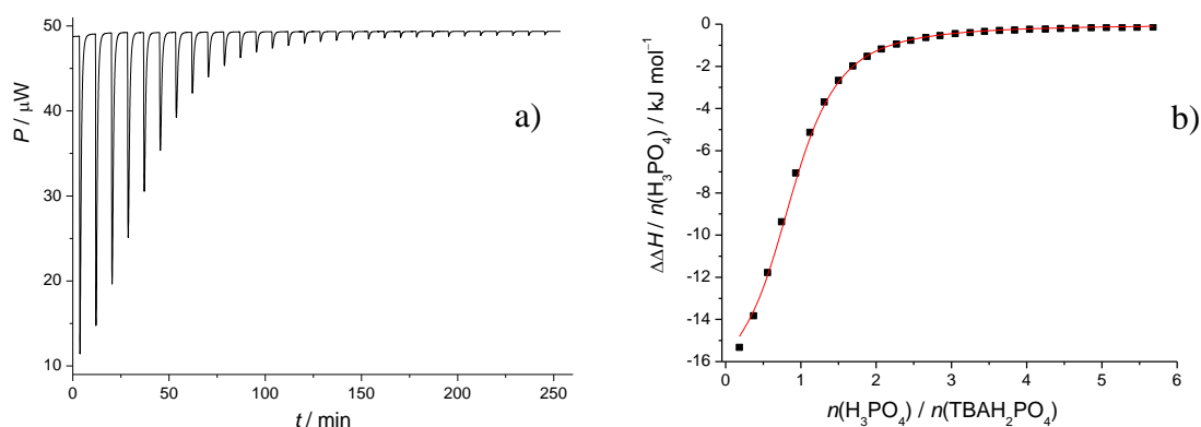
Slika 22. a) Mikrokalorimetrijska titracija otopine TBAH 2 PO 4 ( c = 5,18 \times 10^{-4} \text{ mol dm}^{-3} ) s H 3 PO 4 ( c = 0,0226 \text{ mol dm}^{-3} ) u DMSO pri 25 °C. b) Ovisnost sukcesivne promjene entalpije o množinskom omjeru n(\text{H}_3\text{PO}_4) / n(\text{TBAH}_2\text{PO}_4) ; ■ izmjerene vrijednosti, — izračunane vrijednosti.
