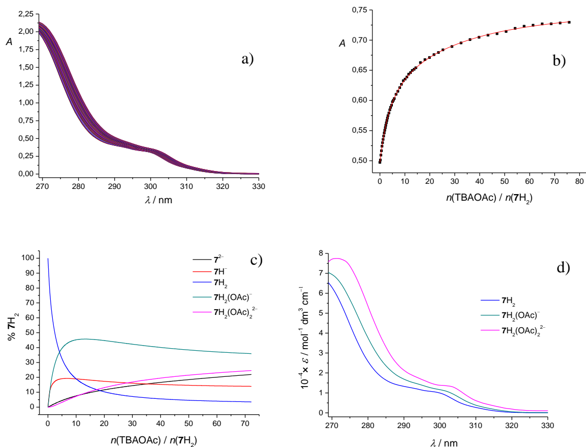
Slika 57. a) Spektrofotometrijska titracija 7\text{H}_2 ( c = 3,03 \times 10^{-5} \text{ mol dm}^{-3} ) s TBAOAc ( c = 5,08 \times 10^{-3} \text{ mol dm}^{-3} ) u DMSO. Spektri su korigirani za razrjeđenje. l = 1 \text{ cm} , (25,0 \pm 0,1) ^\circ\text{C} . b) Ovisnost apsorbancije otopine 7\text{H}_2 pri 285 nm o množinskom omjeru n(\text{TBAOAc}) / n(7\text{H}_2) . ■ izmjerene vrijednosti, — izračunane vrijednosti. c) Distribucija pojedinih vrsta tijekom titracije otopine 7\text{H}_2 s TBAOAc. d) Karakteristični UV spektri spoja 7\text{H}_2 i njegovih kompleksa s acetatom.
