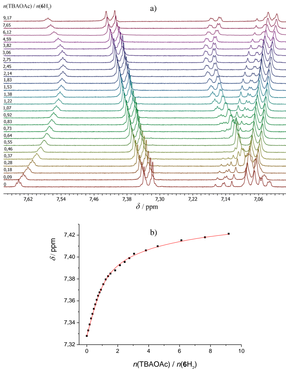
Slika 60. a) ^1\text{H} NMR titracija 6\text{H}_2 ( c = 6,05 \times 10^{-4} \text{ mol dm}^{-3} ) s TBAOAc ( c = 9,71 \times 10^{-3} \text{ mol dm}^{-3} ) u \text{DMSO-}d_6 pri (25,0 \pm 0,1) \text{ }^\circ\text{C} . b) Ovisnost kemijskog pomaka \text{H}_a protona tijekom ^1\text{H} NMR titracije s TBAOAc o množinskom omjeru n(\text{TBAOAc}) / n(6\text{H}_2) . ■ izmjerene vrijednosti, — izračunane vrijednosti.
