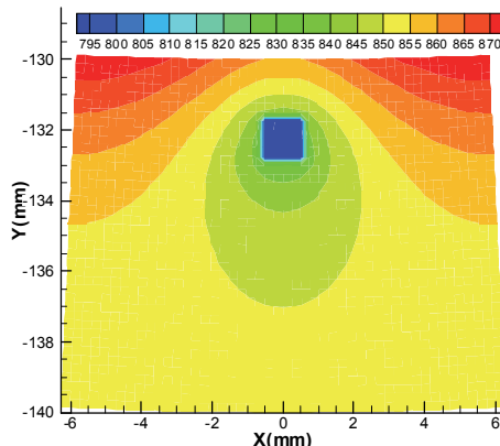
图 6 冷却结构出口截面温度计算值分布
