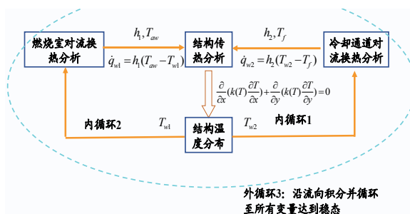
图 1 燃烧室一维分析示意图
