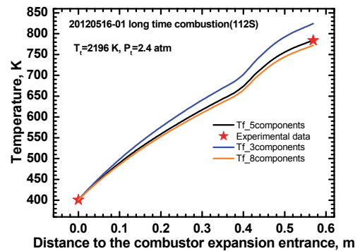
图 8 三、五、八组分替代模型计算油温与测量油温
