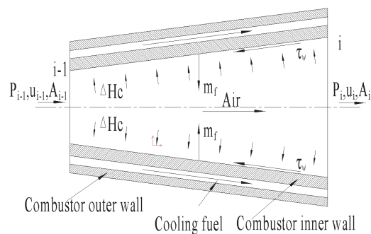
图 2 燃烧室一维分析示意图
