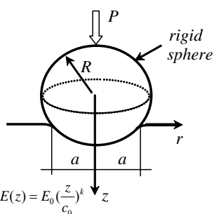
图 1 三维黏附接触模型
