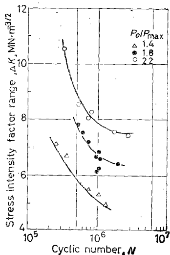
图 1 不同过载比的 \Delta K-N 曲线 Fig. 1 \Delta K-N curves for various overload ratio
