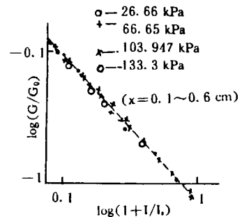
Fig. 4 \log(1 + I/I_s) \sim \log(G/G_0)
