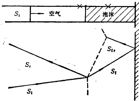
图1 实验装置示意图与流动波图 ×为测压点
